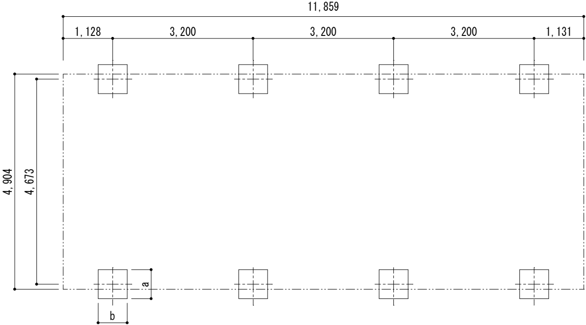
■基礎配置図
